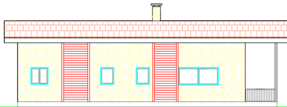
ALZADO POSTERIOR
